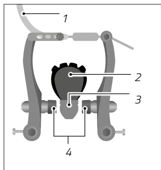
Sl.: Mehanske zavora na obroču (na podlagi primera)
