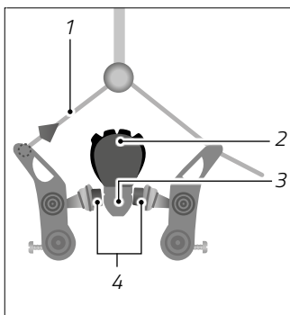
Sl.: Mehanske zavora na obroču (na podlagi primera)
