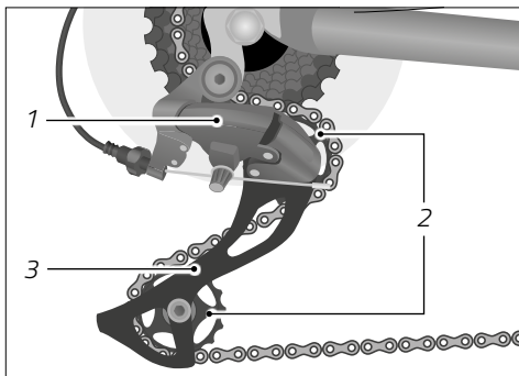
Sl.: Premični sestavni deli verižnega menjalnika (na podlagi primera)
